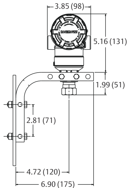
Figura 21: Configuraciones de montaje típicas del Rosemount 2051T con soporte de montaje opcional
