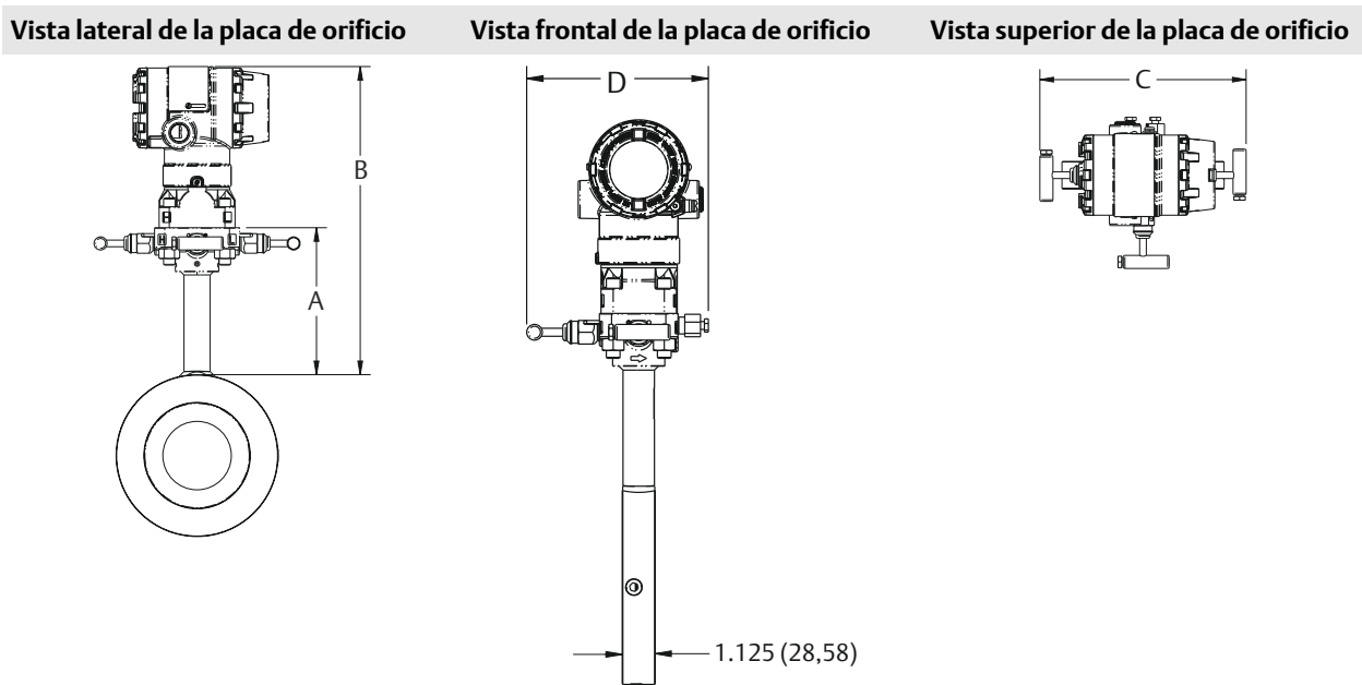
Placa de orificio compacta (tipo de placa de orificio código P)
