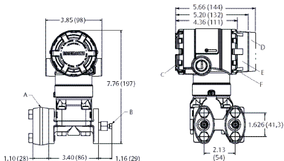
Figura 10: Rosemount 2051C Coplanar con brida tradicional
