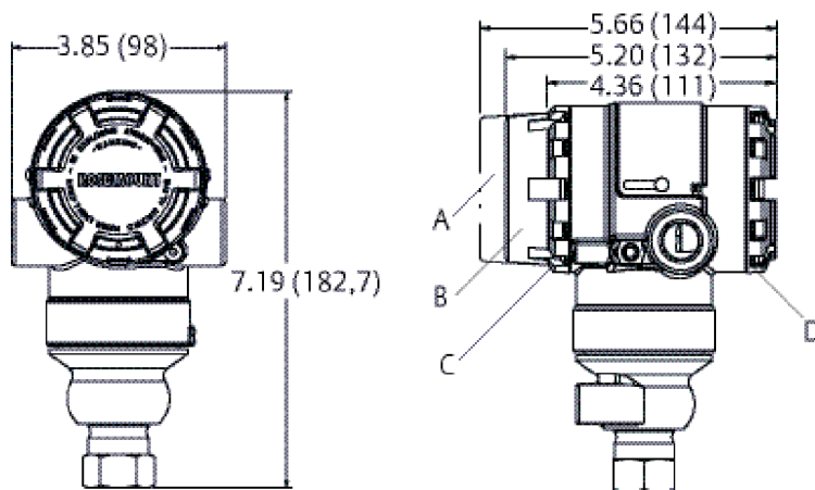
Figura 13: Rosemount 2051T
