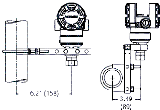
Figura 21: Configuraciones de montaje típicas del Rosemount 2051T con soporte de montaje opcional
