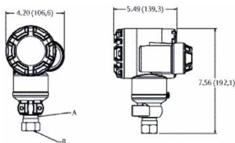
Figura 19: Carcasa de Rosemount 2051 Inalámbrico con plataforma In-line
