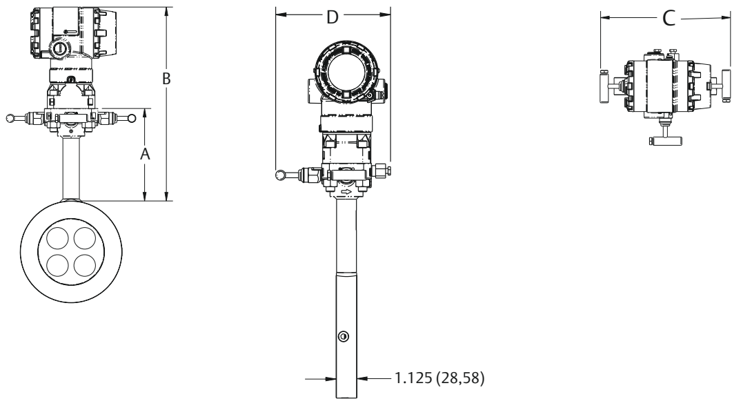
Placa de orificio compacta (tipo de placa de orificio código P)
